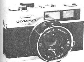
Olympus 35 DC lommekamera Lysstærkt kompaktkamera med avanceret programmering fra 1/15 sek. bl. 1,7 til 1/500 sek. bl. 16, kontrolknop for modlys og angivelse af tid og blænder i lysrammesøgeren. Koblet afstands-måler, selvudløser, blitzautomatik, batteritest. Ekstra skarptegnende Olympus-objektiv F. Zuiko 1,7/40 mm 6-linset.
