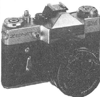
Zenit EM Enøjet spejlreflekskamera med indbygget lysmåler. Microprismesøger. Springblændeautomatik. Lukkertider fra 1 til 1/500 sek + B. Selvudløser. Objektivprogram fra 37 mm til 1000 mm.
