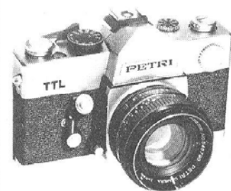
Petri TTL SLR-systemkamera med krydskoblet CdS-måling gennem objektivet. Spaltelukker 1-1/1000 sek. + B. Standardgevind. Med objektiv 1,8/55 mm.
